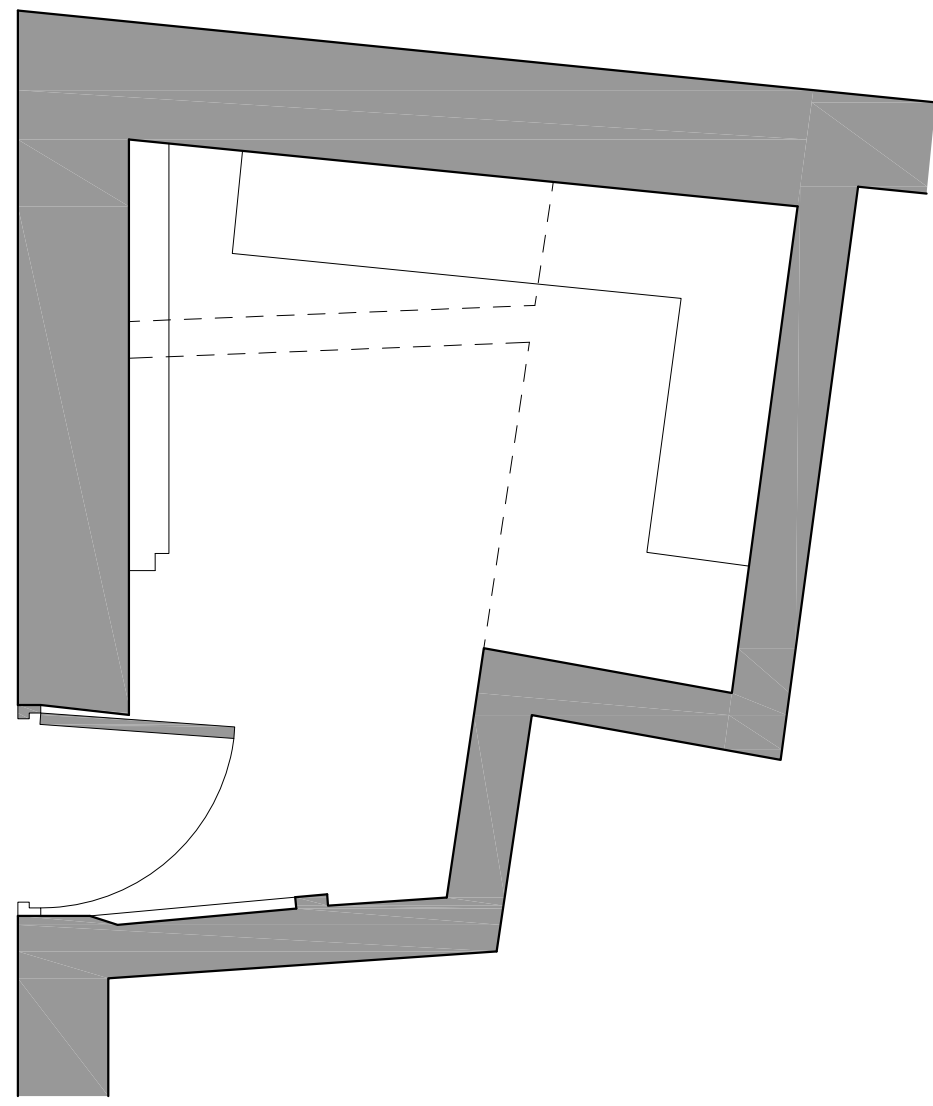
Planta nivel +1,00
