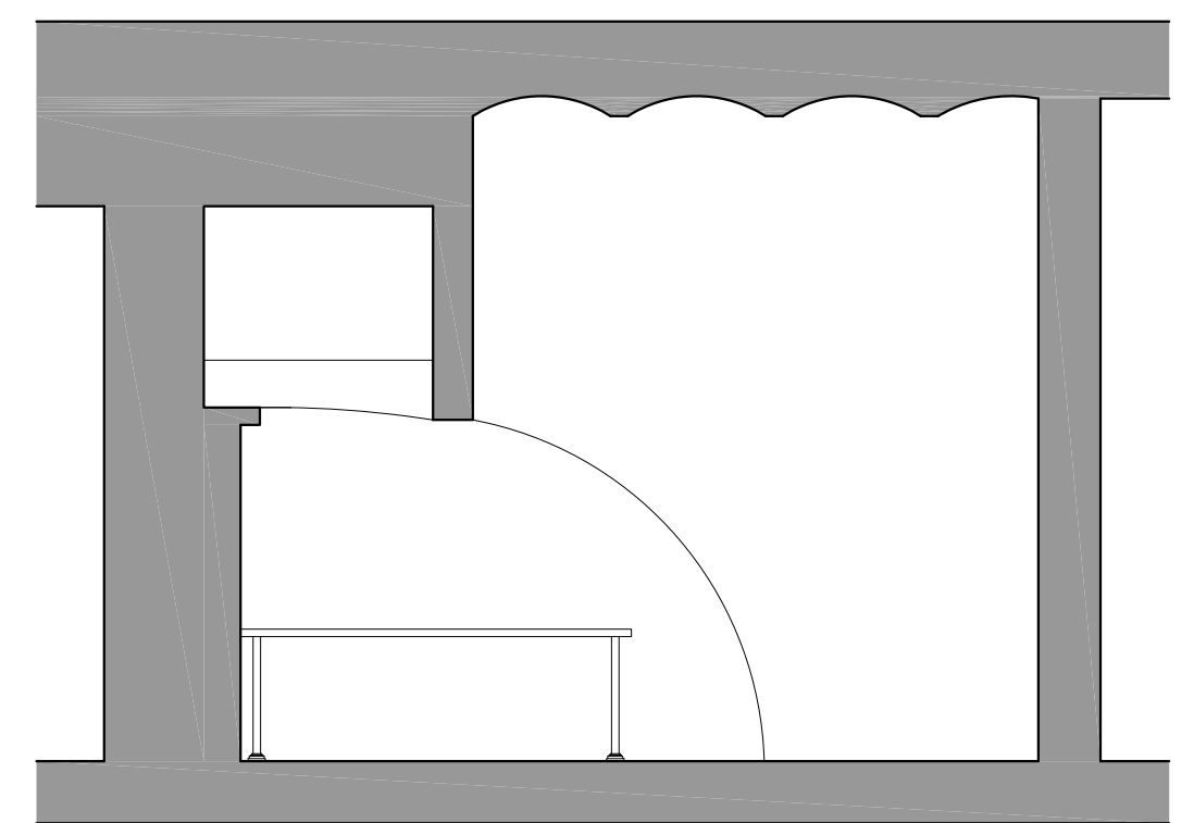
Sección B
